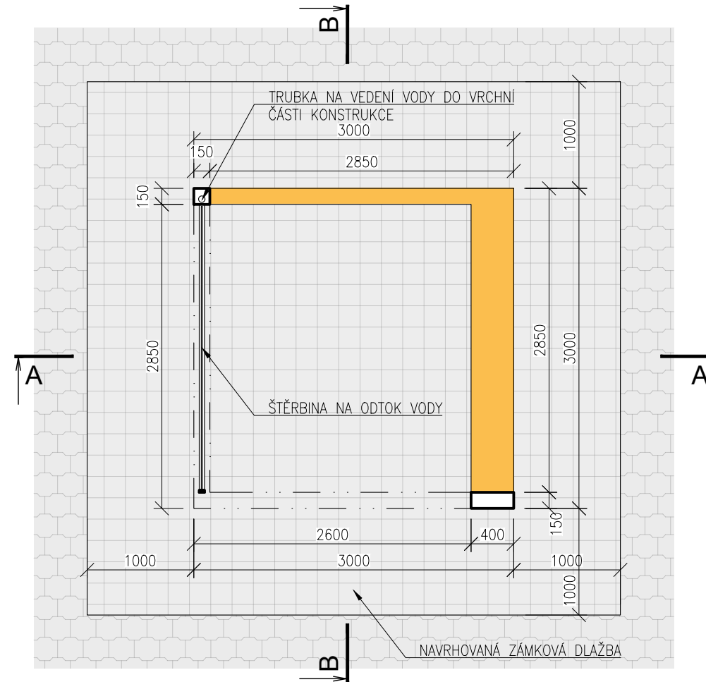
PŮDORYS
