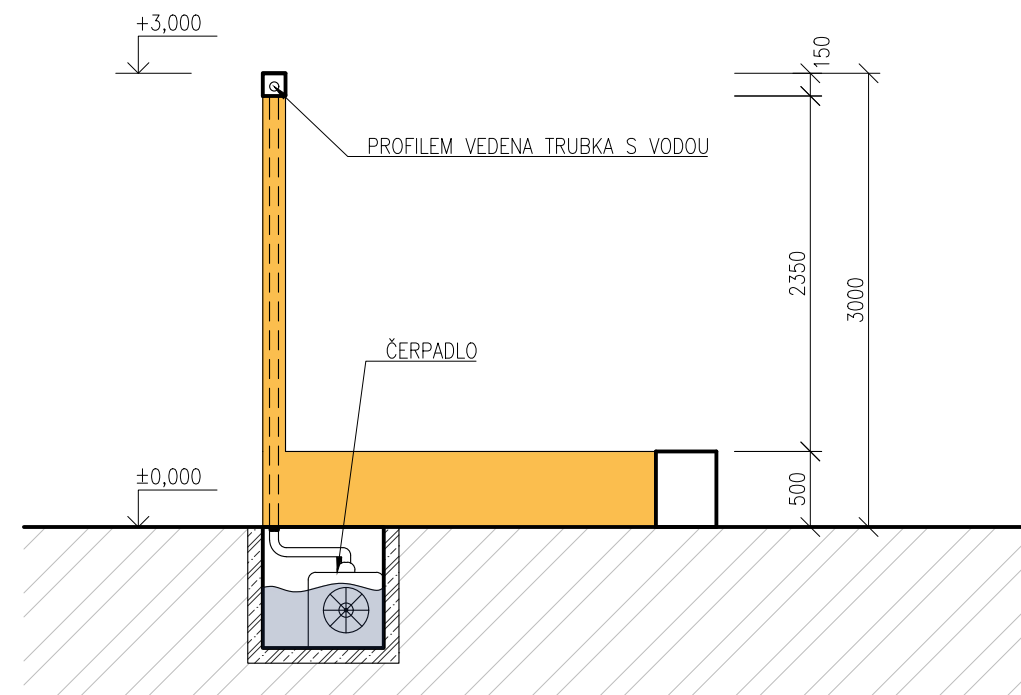
ŘEZ A
